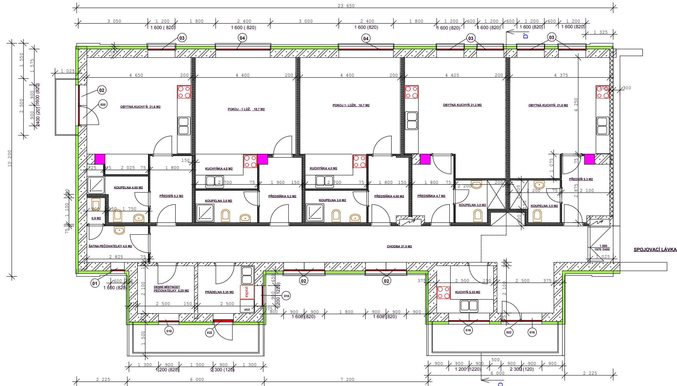
PŮDORYS 1.PATRA - zadní pavilon - dětské oddělení
