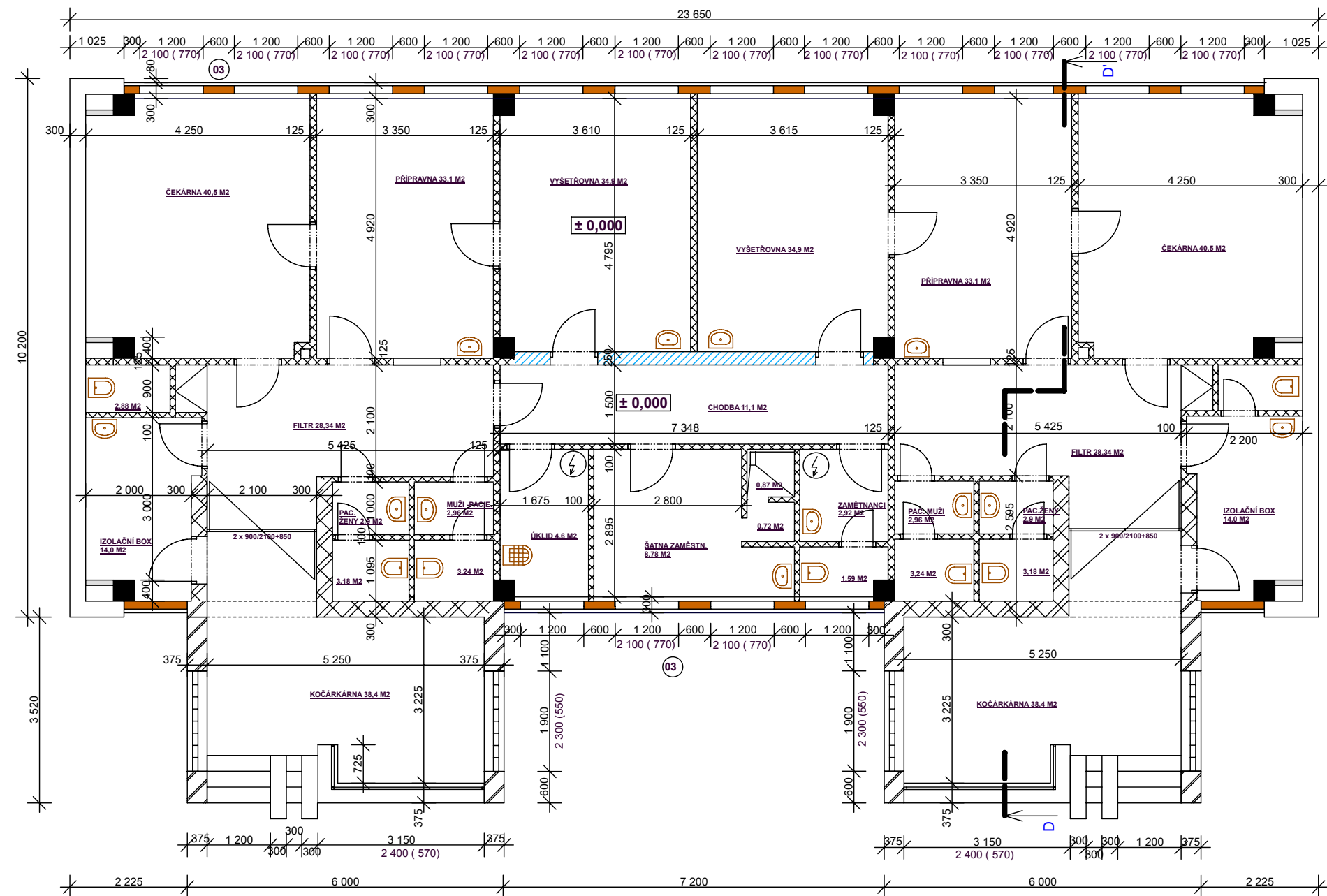
PŮDORYS PŘÍZEMÍ - zadní pavilon - dětské oddělení
