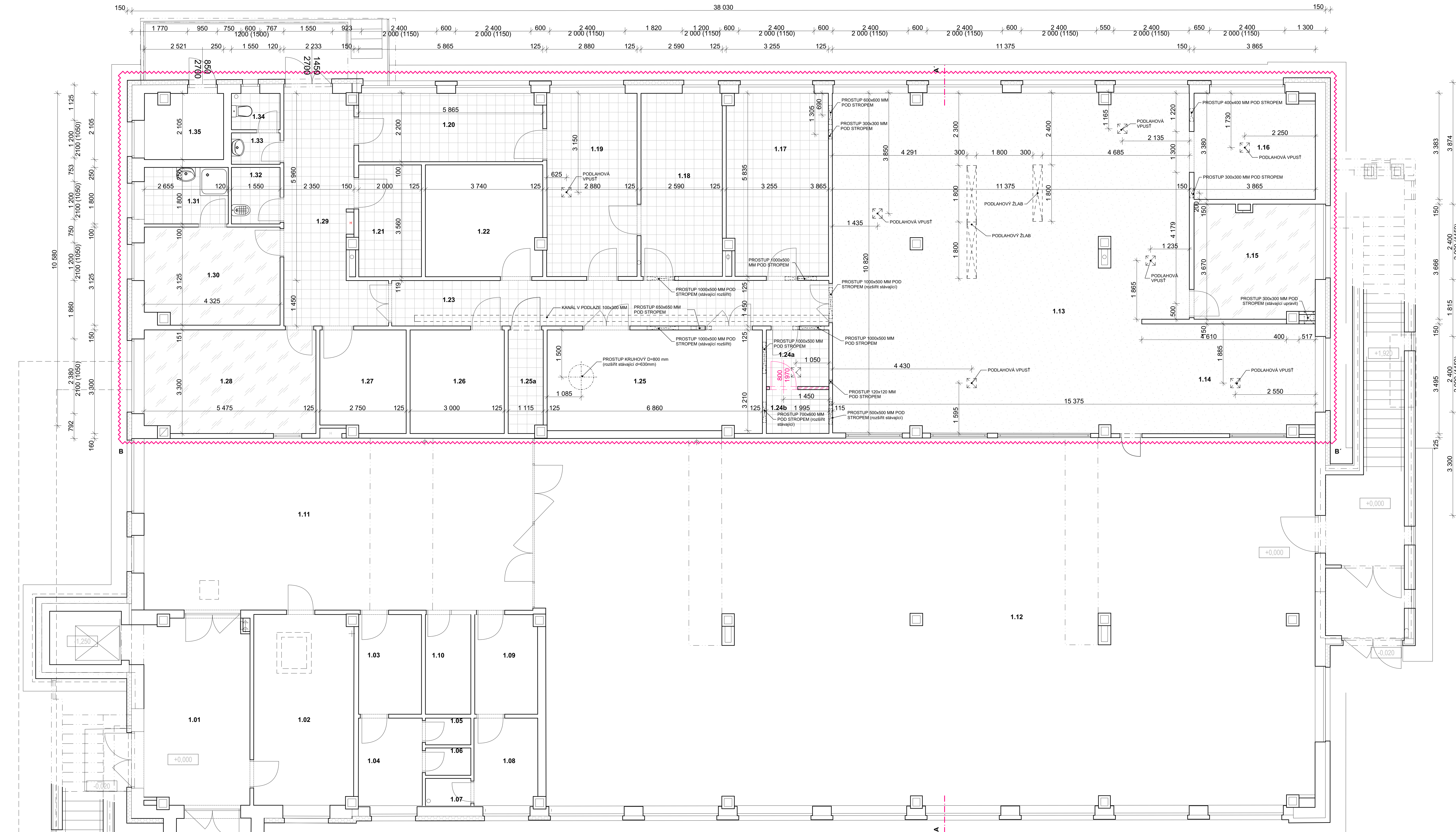
LEGENDA MÍSTNOSTÍ - nový stav
